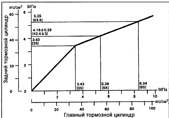
График работы регулятора давления (модели до 1996 г.).
