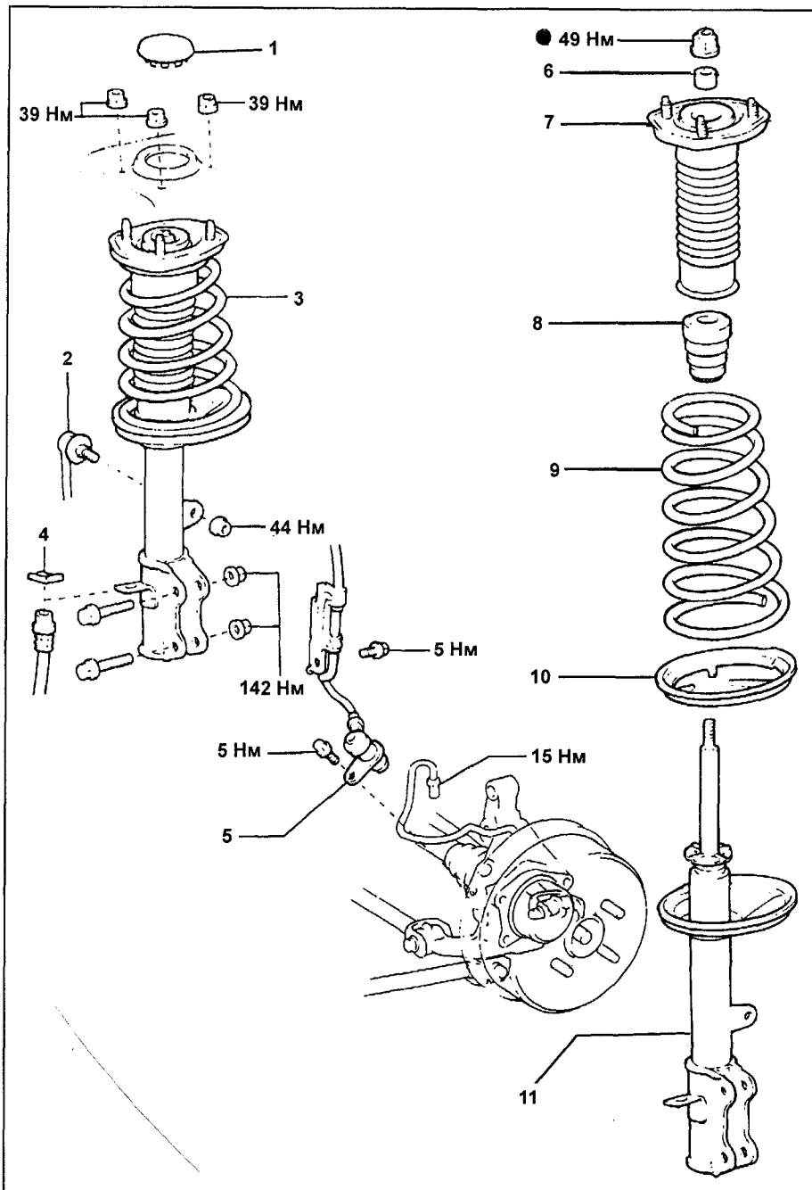
Стойка задней подвески. 1 - крышка, 2 - стойка стабилизатора поперечной устойчивости, 3 - стойка задней подвески в сборе, 4 - фиксатор, 5 - датчик частоты вращения (ABS), 6 - втулка, 7 - верхняя опора стойки, 8 - ограничитель хода сжатия, 9 - пружина, 10 - нижнее седло пружины, 11 - стойка задней подвески.
