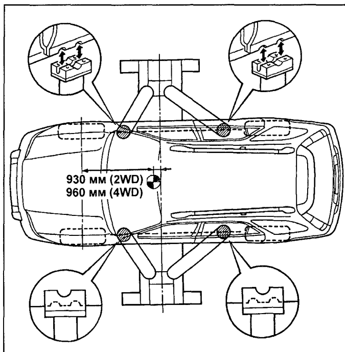
Точки установки лап подъемника.
