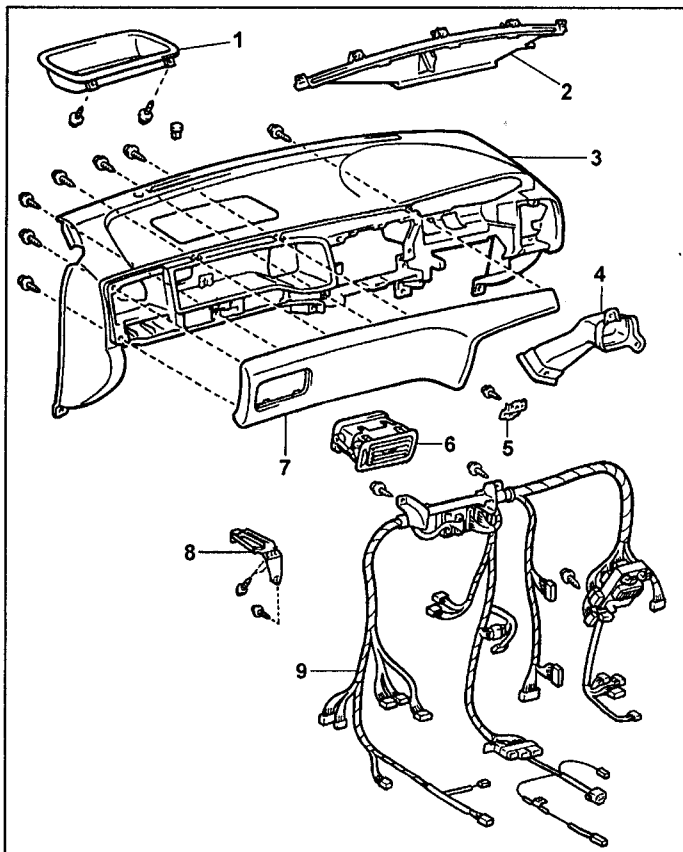
Снятие и установка панели приборов (тип 1).
