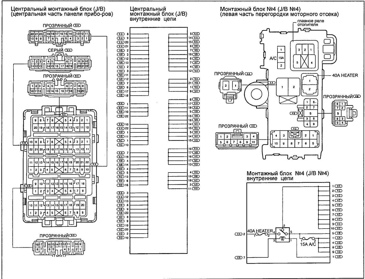
Монтажный блок №4 (J/B №4) (левая часть перегородки моторного отсека)
