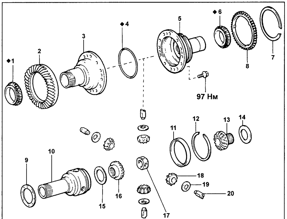
Вал ведущей шестерни главной передачи. 1 - конический роликовый подшипник, 2 - ведущая шестерня главной передачи, 3 - левая чашка ведущей шестерни главной передачи, 4 - кольцевое уплотнение, 5 - правая чашка ведущей шестерни главной передачи, 6 - подшипник, 7 - стопорное кольцо, 8 - ведущая шестерня масляного насоса, 9 - упорная шайба, 10 - межосевой дифференциал, 11 - распорная втулка, 12 - стопорное кольцо, 13 - полуосевая шестерня межосевого дифференциала, 14 - коническая пружинная шайба, 15 - упорная шайба, 16 - полуосевая шестерня межосевого дифференциала, 17 - держатель осей сателлитов, 18 - сателлит межосевого дифференциала, 19 - упорная шайба сателлита межосевого дифференциала, 20 - ось сателлитов межосевого дифференциала.
