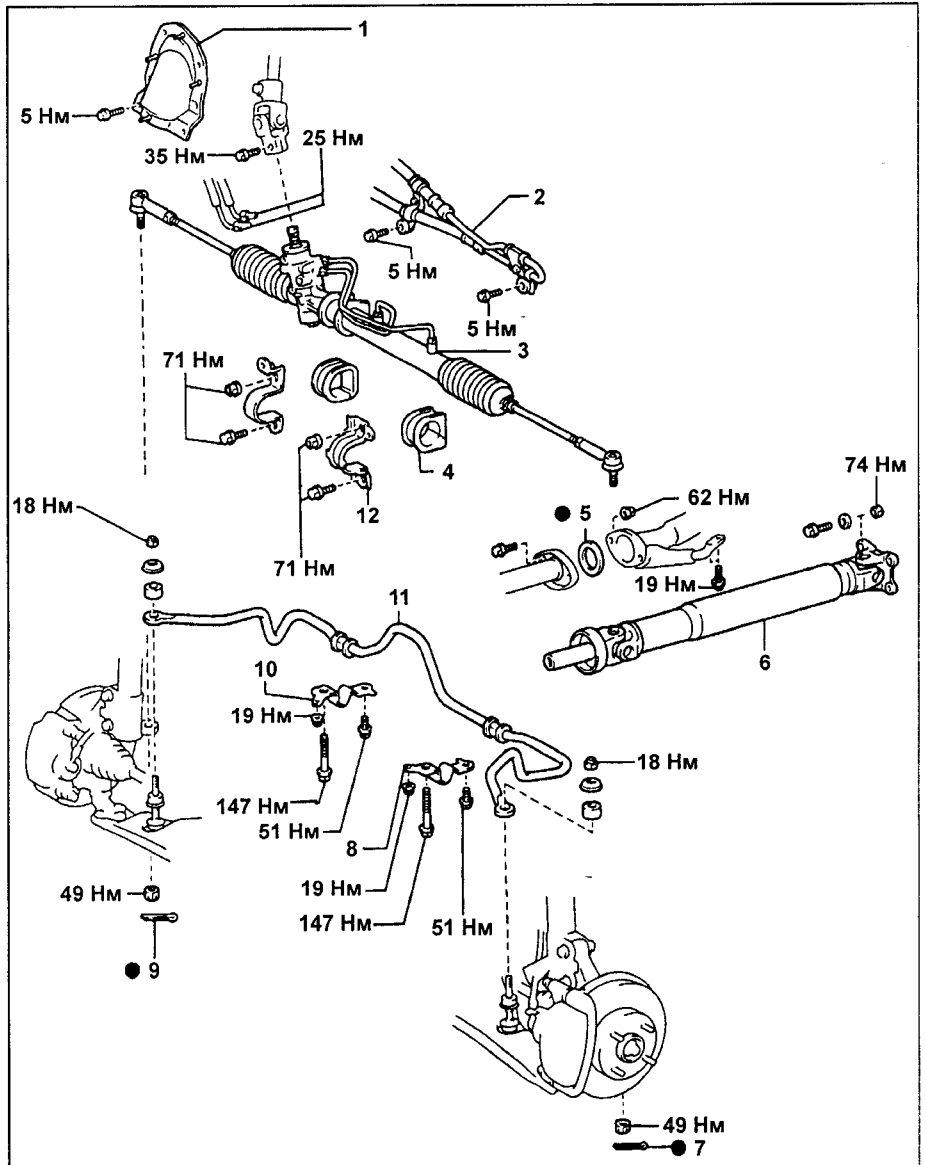
Снятие рулевого механизма. 1 - крышка, 2 - нагнетательный трубопровод (7A-FE), 3 - рулевой механизм в сборе, 4 - втулка, 5 - прокладка, 6 - карданный вал, 7, 9 - шплинт, 8, 10 - кронштейн крепления стабилизатора поперечной устойчивости, 11 - стабилизатор поперечной устойчивости, 12 - кронштейн крепления рулевого механизма.
