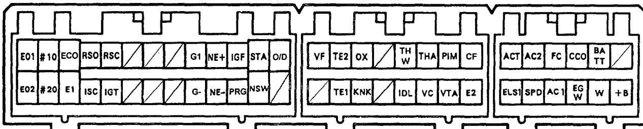
4A-FE (с 1995 г)
