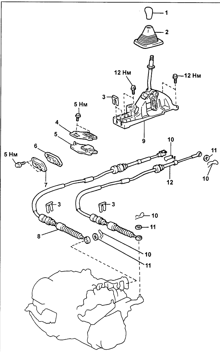
Рычаг переключения передач. 1 - рукоятка рычага переключения передач, 2 - чехол, 3 - фиксатор, 4 - держатель уплотнения №1, 5 - уплотнение №1, 6 - держатель уплотнения №2, 7 - уплотнение №2, 8 - трос переключения передач, 9 - рычаг переключения передач в сборе, 10 - шплинт, 11 - шайба, 12 - трос выбора передач.
