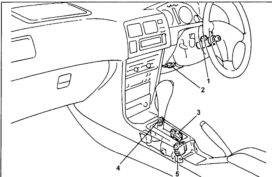
Система блокирования селектора. 1 - электромагнитный клапан блокировки ключа зажигания, 2 - выключатель стоп-сигналов, 3 - узел системы блокировки селектора, 4 - выключатель разблокировки селектора, 5 - электронный блок управления блокировкой селектора.
