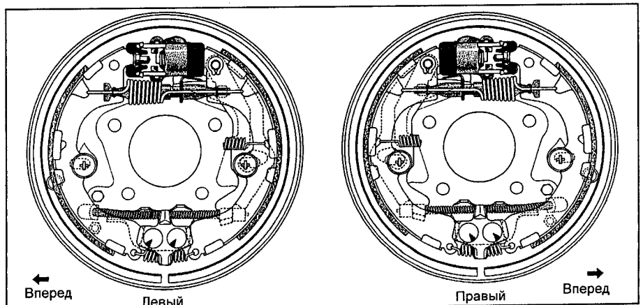
Схема установки деталей задних барабанных тормозов (модели с 1996 г.).
