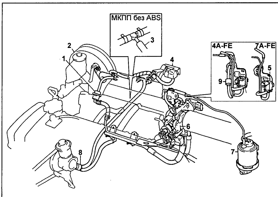
Схема вакуумных линий (4A-FE, 7A-FE). 1 - регулятор давления топлива, 2 - вакуумный усилитель тормозов, 3 - к сервоприводу трансмиссии, 4 - датчик абсолютного давления во впускном коллекторе, 5 - электропневмоклапан системы улавливания паров топлива, 6 - корпус дроссельной заслонки, 7 - аккумулятор паров топлива, 8 - клапан системы управления подачей воздуха (подачи дополнительного воздуха), 9 - обратный клапан (4A-FE до 1997 г).
