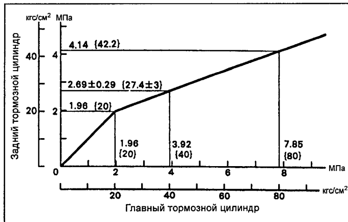
График работы регулятора давления (модели 2WD с 1996 г. (4A-FE)).
