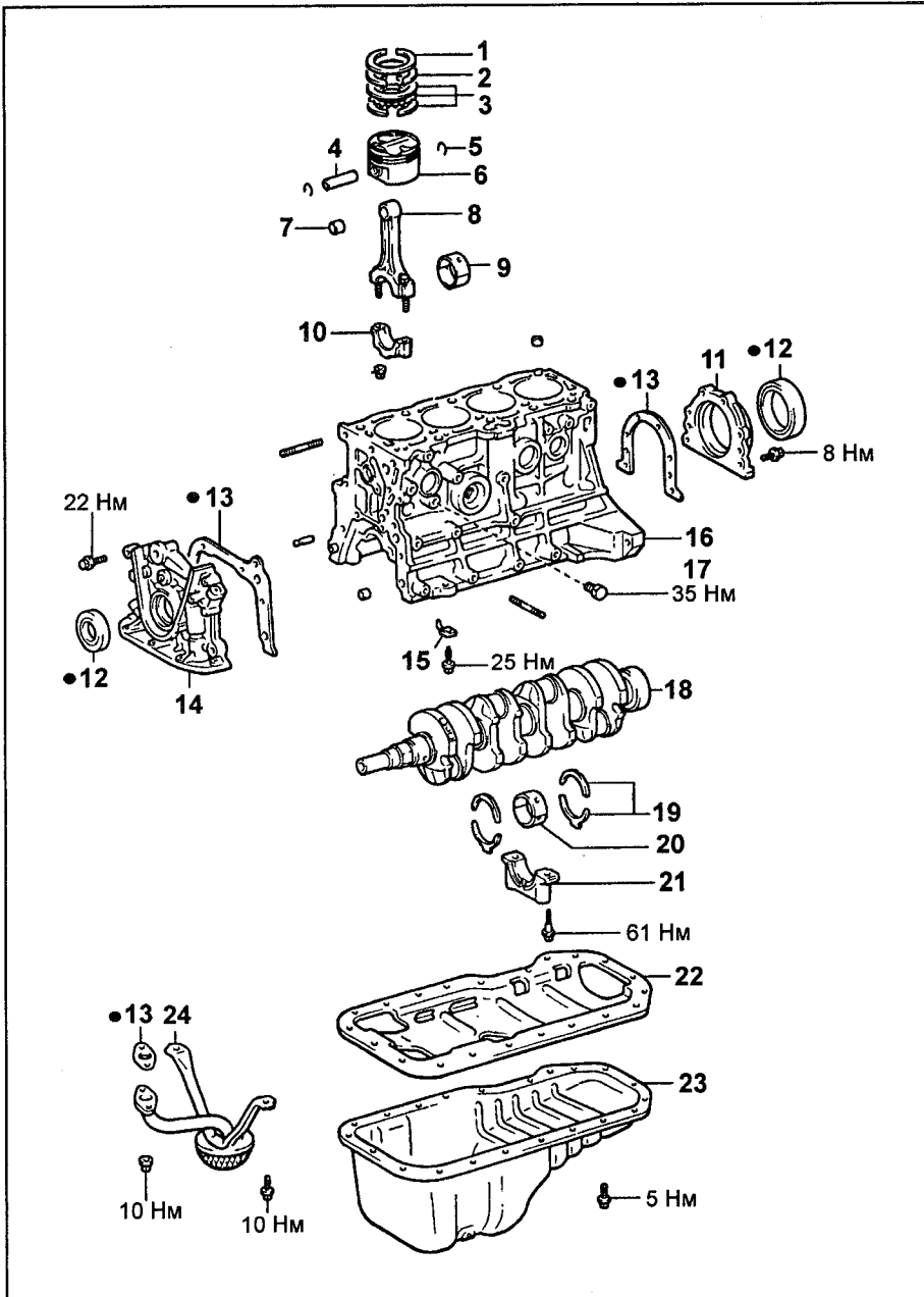
Блок цилиндров (4A-GE). 1 - верхнее компрессионное кольцо, 2 - нижнее компрессионное кольцо, 3 - маслосъемные кольца с расширителем, 4 - поршневой палец, 5 - стопорное кольцо, 6 - поршень, 7 - втулка верхней головки шатуна, 8 - шатун, 9 - вкладыш шатунного подшипника, 10 - крышка шатуна, 11 - держатель сальника, 12 - сальник, 13 - прокладка, 14 - масляный насос в сборе, 15 - масляная форсунка, 16 - блок цилиндров, 17 - пробка слива охлаждающей жидкости, 18 - коленчатый вал, 19 - упорные полукольца, 20 - вкладыш коренного подшипника, 21 - крышка коренного подшипника, 22 - маслоуспокоитель, 23 - масляный поддон, 24 - маслоприемник.
