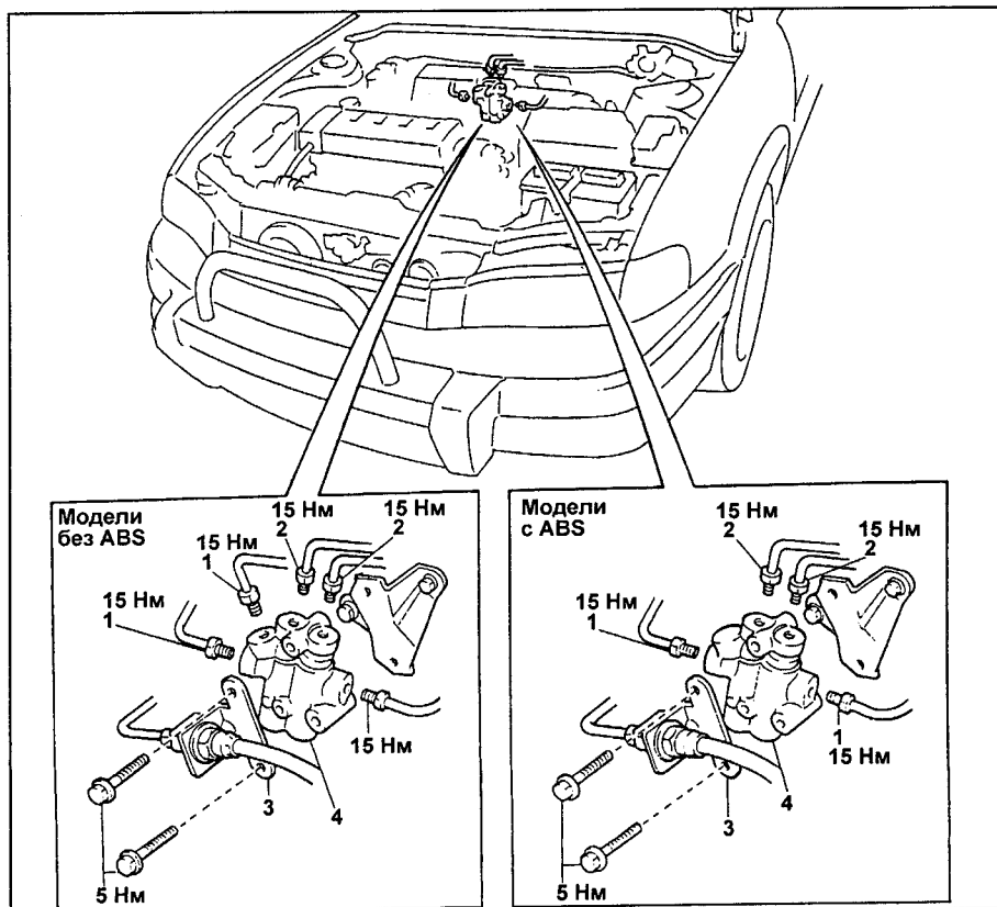
Снятие регулятора давления. 1 - трубка передних тормозов, 2 - трубка задних тормозов, 3 - кронштейн (МКПП), 4 - регулятор давления.
