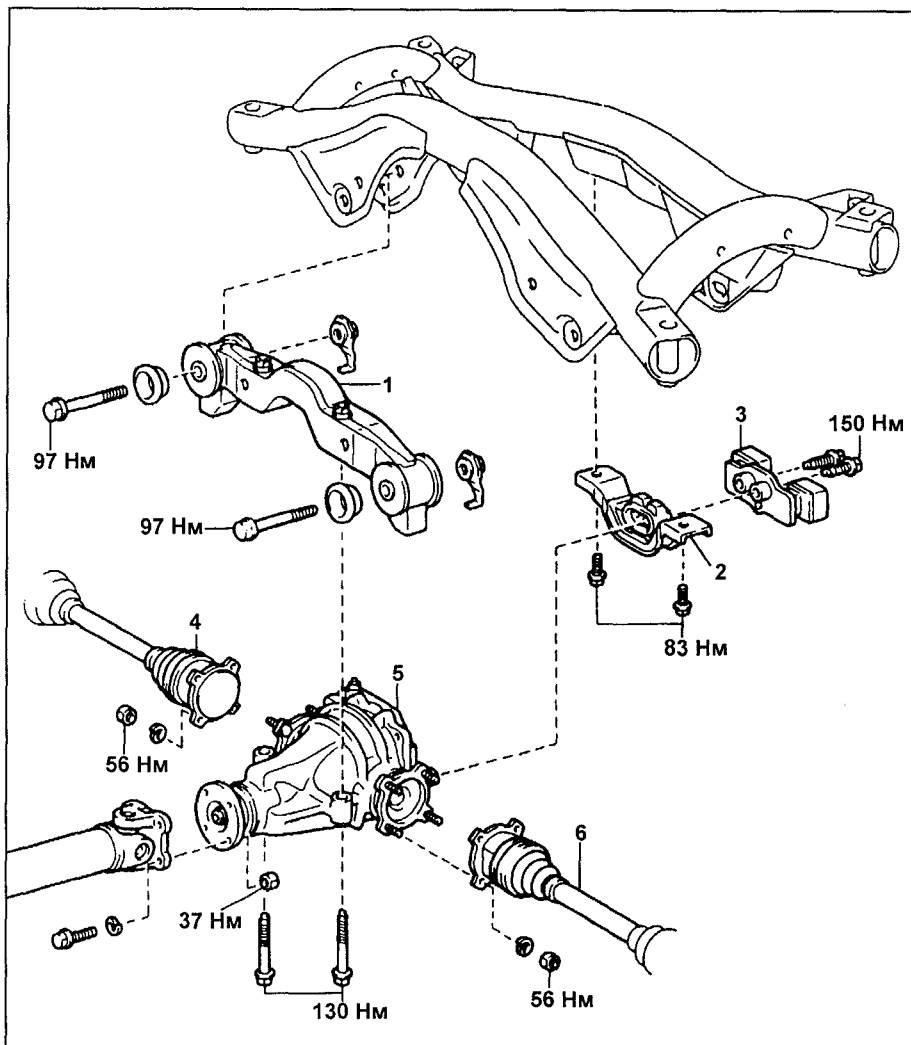
Снятие редуктора заднего моста. 1 - передняя опора редуктора, 2 - задняя опора редуктора, 3 - демпфер (модели с МКПП), 4 - правый приводной вал, 5 - редуктор заднего моста в сборе, 6 - левый приводной вал.
