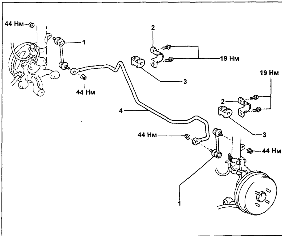
Снятие стабилизатора поперечной устойчивости. 1 - стойка стабилизатора, 2 - кронштейн крепления стабилизатора, 3 - втулка, 4 - стабилизатор поперечной устойчивости.
