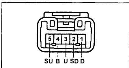
Передние двери, задние двери (тип 1)
