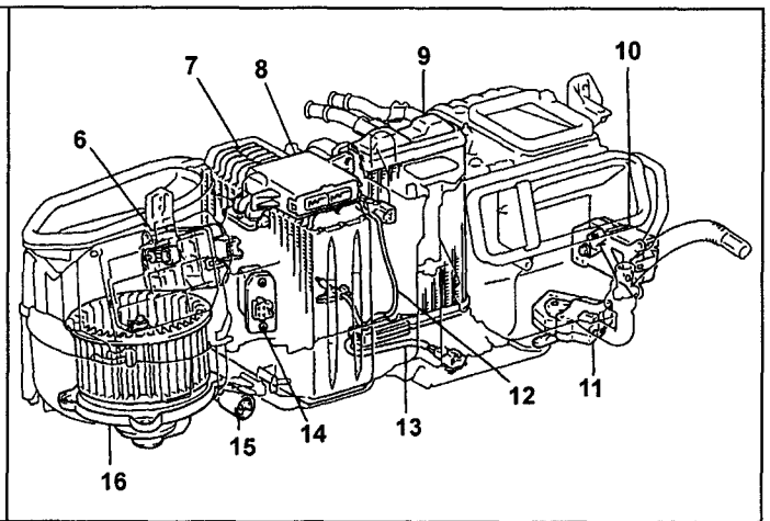
Передний блок системы отопителя и системы кондиционирования воздуха в сборе.
