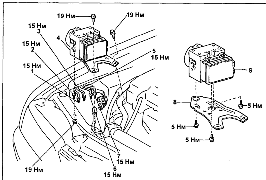
Снятие модулятора давления (модели с 1996 г.). 1 - трубка №8, 2 - трубка №3, 3 - трубка №13, 4 - модулятор давления в сборе с кронштейном, 5 - трубка №1, 6 - трубка №6, 7 - трубка №7, 8 - кронштейн, 9 - модулятор давления.
