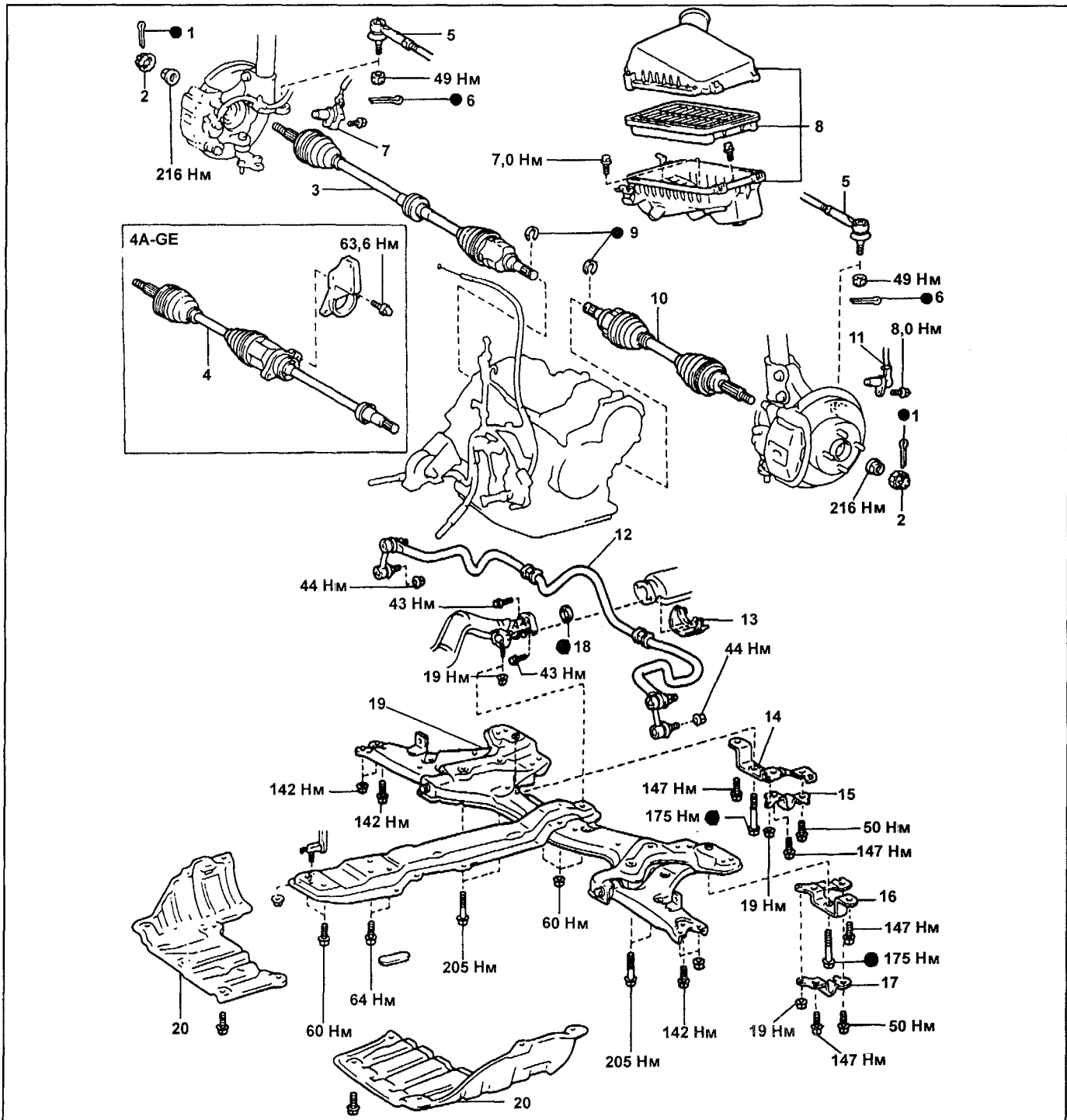
Снятие коробки передач в сборе. 1 - шплинт, 2 - контргайка, 3, 4 - приводной вал, 5 - наконечник рулевой тяги, 6 - шплинт, 7 - датчик частоты вращения, 8 - воздушный фильтр в сборе, 9 - стопорное кольцо, 10 - приводной вал, 11 - датчик частоты вращения, 12 - стабилизатор поперечной устойчивости, 13 - передний кронштейн выхлопной трубы, 14, 16 - кронштейн нижнего рычага подвески, 15, 17 - кронштейн №1 рычага стабилизатора, 18 - прокладка, 19 - поперечная балка в сборе с нижними рычагами подвески, 20 - нижний кожух защиты.
