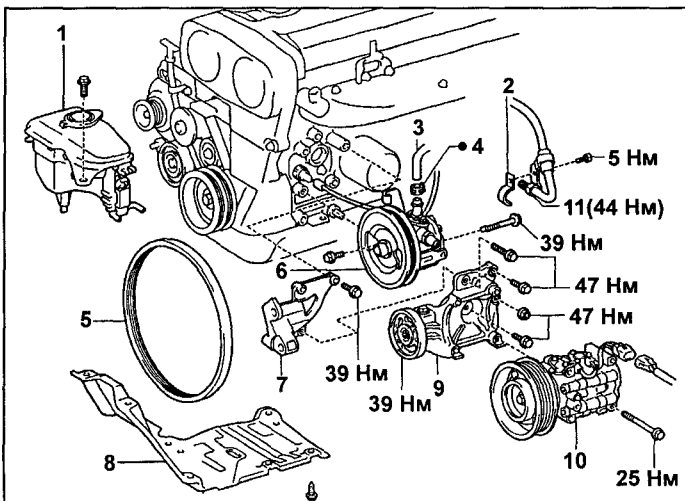
Снятие насоса усилителя рулевого управления (4A-GE). 1 - бачок омывателя, 2 - кронштейн нагнетательного трубопровода, 3 - возвратный трубопровод, 4 - хомут, 5 - приводной ремень, 6 - насос усилителя рулевого управления в сборе, 7 - кронштейн крепления насоса, 8 - нижний защитный кожух двигателя, 9 - ролик натяжителя в сборе с кронштейном, 10 - компрессор кондиционера, 11 - нагнетательный трубопровод.
