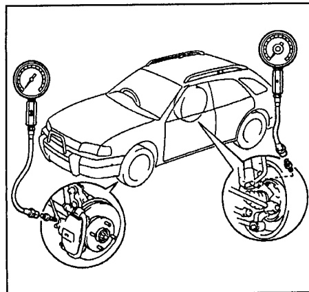
Проверка давления жидкости.
