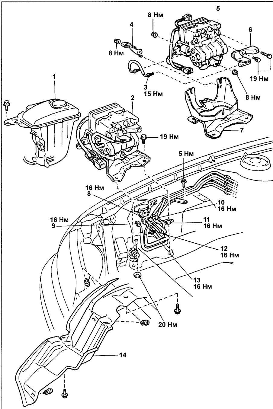
Снятие модулятора давления (модели до 1996 г.). 1 - бачок омывателя, 2 - модулятор давления в сборе с кронштейном, 3 - трубка модулятора №1, 4 - кронштейн №4, 5 - модулятор давления, 6 - кронштейн №1, 7 - кронштейн модулятора давления, 8 - трубка №6, 9 - трубка №8, 10 - трубка №7, 11 - трубка №1, 12 - трубка №3, 13 - трубка №13, 14 - подкрылок.
