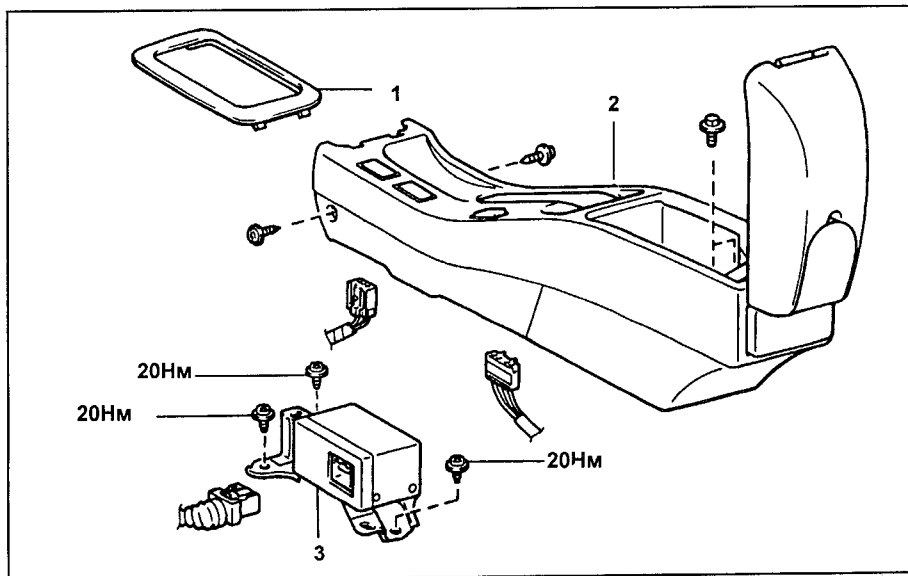
Датчик подушек безопасности (модели с 1996 года). 1 - отделка отверстия под рычаг АКПП, 2 - задняя консоль, 3 - центральный датчик.
