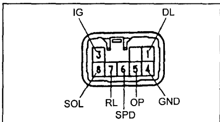
Выводы электронного блока управления блокировкой межосевого дифференциала (4A-FE).
