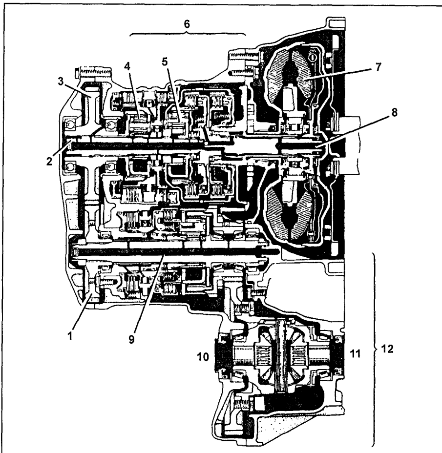
Планетарный механизм коробки передач (А241Н). 1 - ведомая шестерня промежуточной передачи, 2 - промежуточный вал, 3 - ведущая шестерня промежуточной передачи, 4 - задний планетарный ряд, 5 - передний планетарный ряд, 6 - планетарный механизм, 7 - гидротрансформатор, 8 - входной вал, 9 - вал ведущей шестерни главной передачи, 10 - приводной вал, 11 - приводной вал, 12 - дифференциал.
