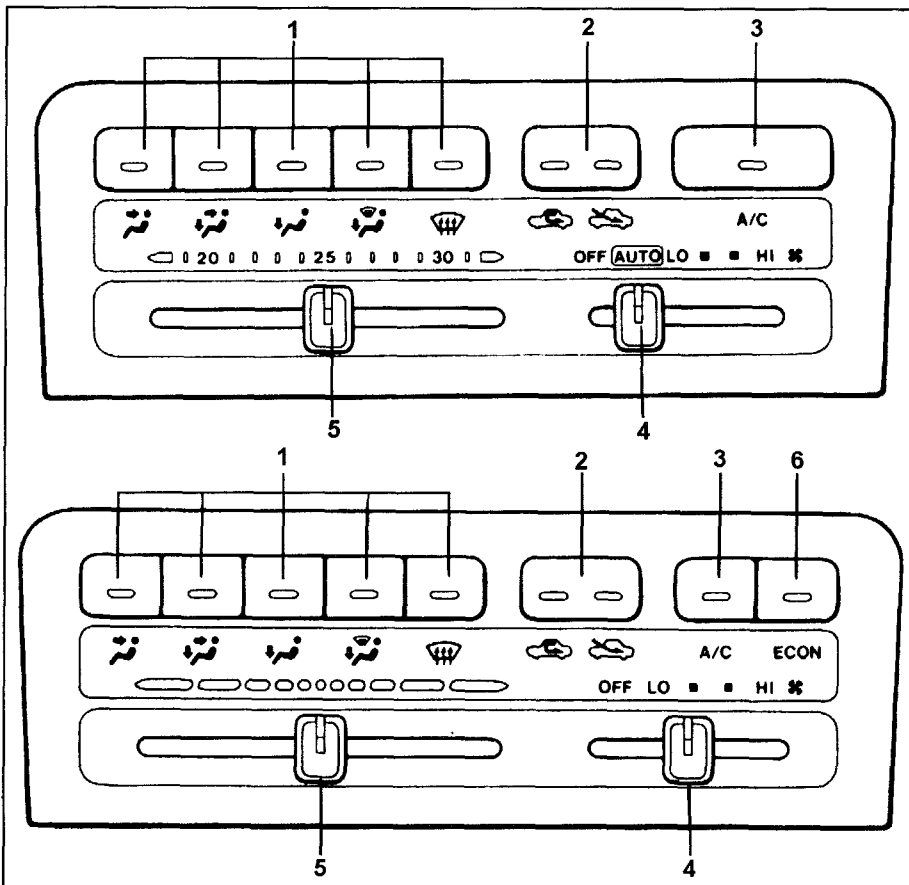
Возможные панели управления отопителем и кондиционером. 1 - панель управления направлением потока воздуха, 2 - рычажок регулировки забора воздуха (вентиляция/рециркуляция), 3 - выключатель кондиционера, 4 - рычажок управления силой потока воздуха, 5 - рычажок регулятора температуры, 6 - выключатель экономичной работы кондиционера.
