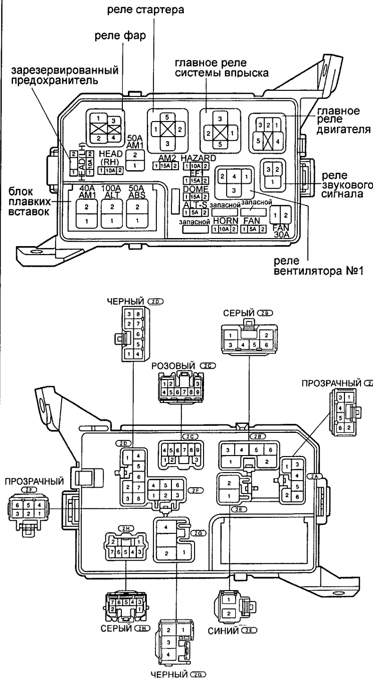
Монтажный блок №2 (J/B №2) и блок плавких вставок (левая часть моторного отсека)
