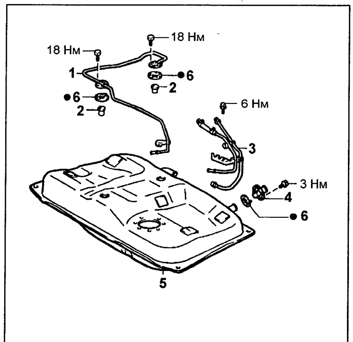
4A-GE. 1 - резервная линия, 2 - клапан отсечки топлива, 3 - трубка возврата топлива, 4 - переходник, 5 - топливный бак, 6 - прокладка.
