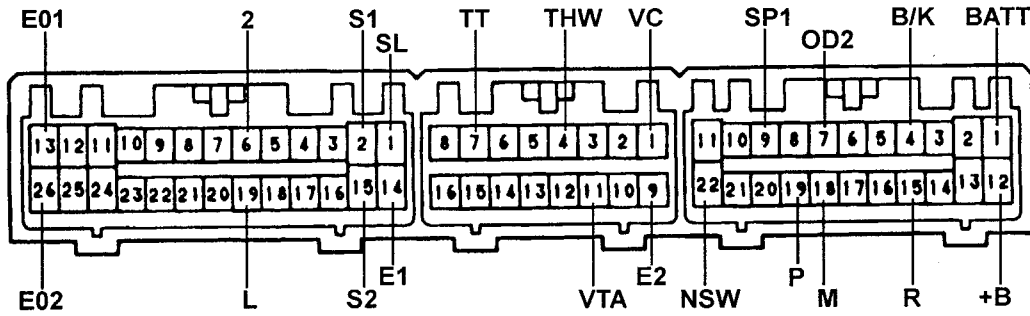
4A-GE (A245E, A246E).
