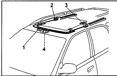
Электропривод люка. 1 - реле управления люком, 3 - правый трос, 4 - левый трос, 4 - электропривод люка.
