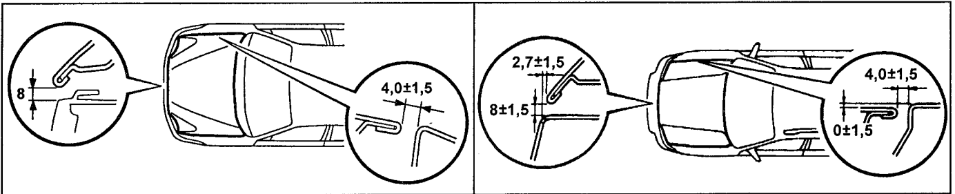
Регулировка зазора между капотом и кузовом автомобиля.
