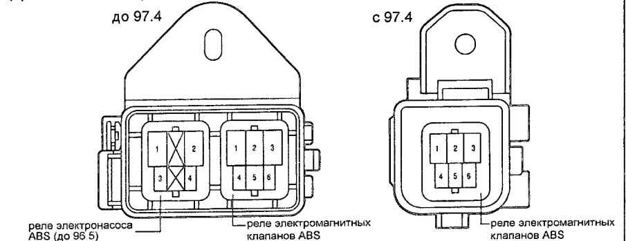
Блок реле ABS (правая часть моторного отсека)
