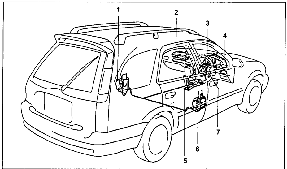
Система безопасности (модели с 1997 года) 1 - преднатяжитель левого ремня безопасности, 2 - подушка безопасности пассажира, 3 - накладка рулевого колеса, 4 - комбинация приборов (индикатор SRS), 5 - центральный датчик системы безопасности, 6 - преднатяжитель ремня безопасности водителя, 7 - спиральный провод.
