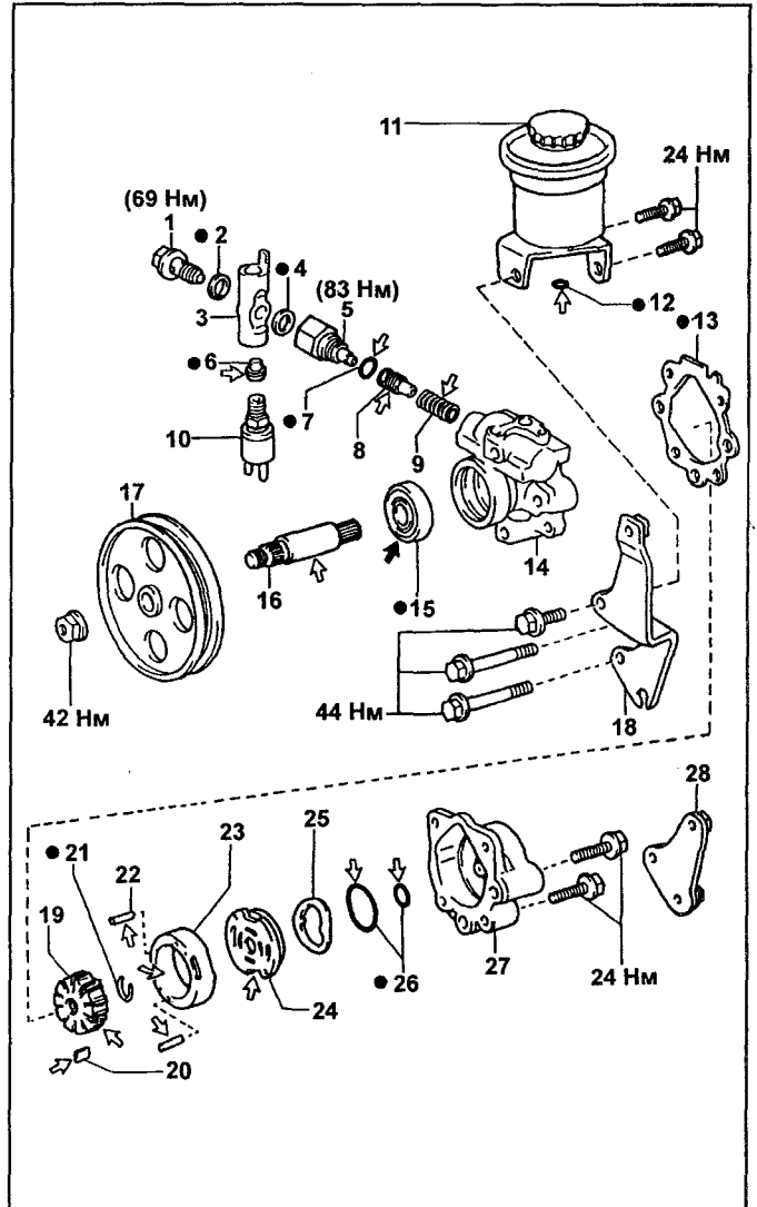
Насос усилителя рулевого управления (4A-FE, 7A-FE). 1 - штуцерный болт, 2, 4, 13 - прокладка, 3 - переходник штуцера нагнетательного трубопровода, 5 - штуцер нагнетательного трубопровода, 6 - седло штуцера, 7, 12, 26 - кольцевое уплотнение, 8 - регулятор расхода, 9 - пружина, 10 - клапан увеличения частоты вращения холостого хода, 11 - бачок, 14 - корпус насоса, 15 - сальник, 16 - вал насоса, 17 - шкив, 18, 28 - кронштейн, 19 - ротор, 20 - лопасть, 21 - стопорное кольцо, 22 - установочный штифт, 23 - статорное кольцо, 24 - задний диск, 25 - волнистая шайба, 27 - крышка корпуса.
