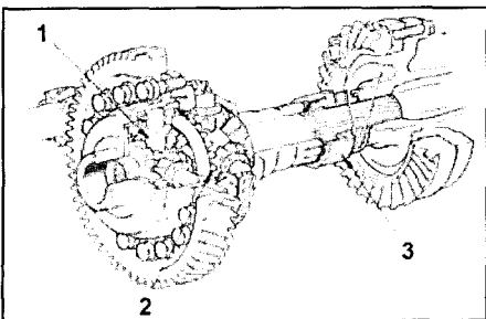
Схема полного привода с механической блокировкой. 1 - межколесный дифференциал, 2 - межосевой дифференциал, 3 - муфта блокировки межосевого дифференциала.
