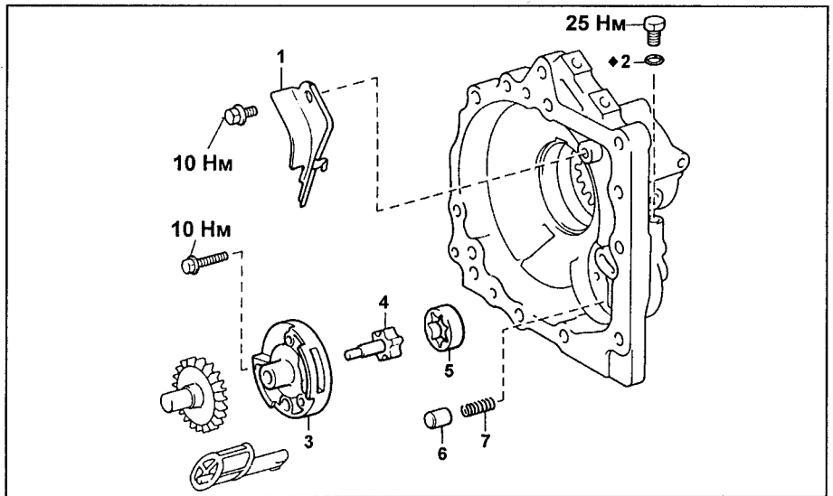
Крышка картера раздаточной коробки. 1 - направляющая пластина шупа, 2 - кольцевое уплотнение, 3 - крышка масляного насоса, 4 - внутренний ротор масляного насоса, 5 - наружный ротор масляного насоса, 6 - перепускной клапан, 7 - пружина.
