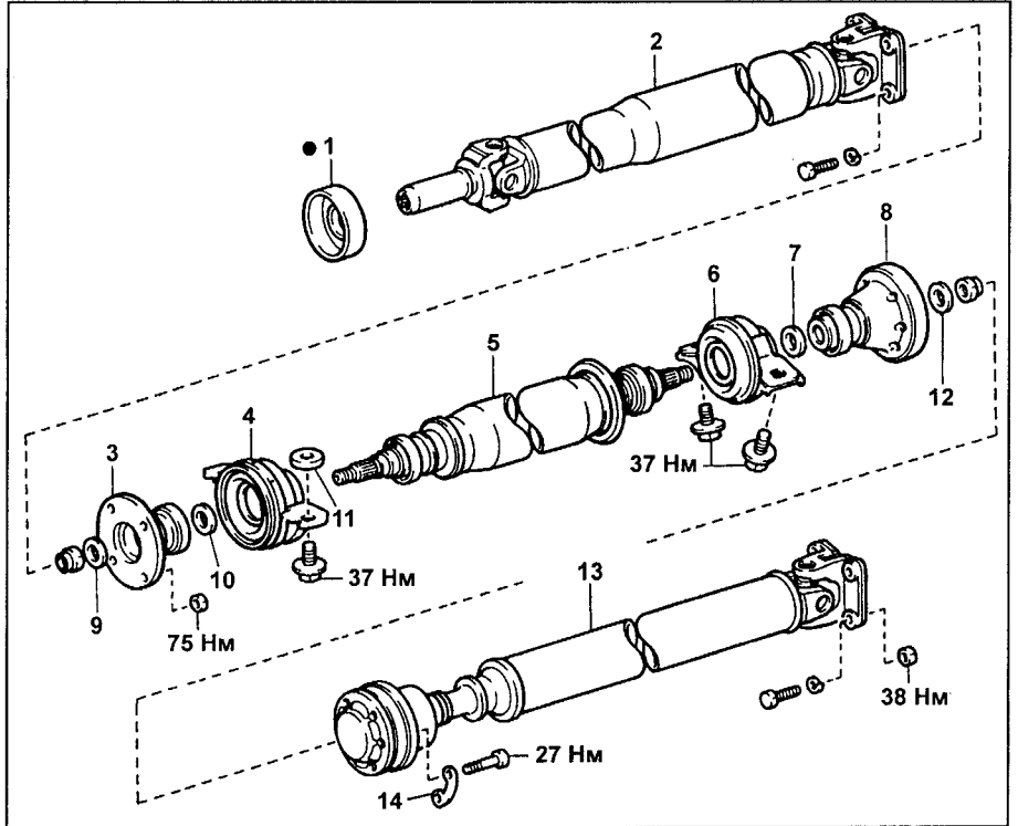
Карданный вал. 1 - пыльник, 2 - передний карданный вал, 3 - передний фланец, 4 - передний опорный подшипник, 5 - промежуточный карданный вал, 6 - задний опорный подшипник, 7, 9, 10 - пластинчатая шайба, 8 - задний фланец, 11 - регулировочная шайба, 12 - шайба, 13 - задний карданный вал, 14 - пластина.
