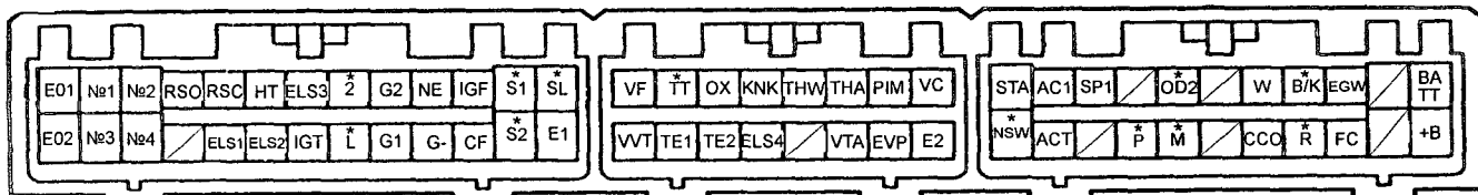
4A-GE (с 1996 г) (* - модели с АКПП)
