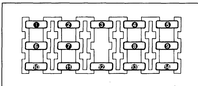
Возможный вариант монтажного блока панели приборов.
