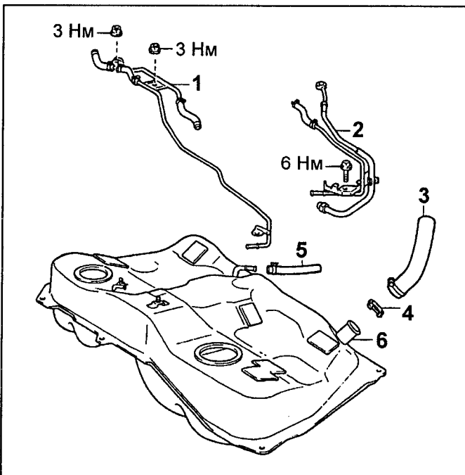
4A-FE, 7A-FE. 1 - резервная линия, 2 - трубка возврата топлива, 3 - топливозаливной шланг, 4 - обратный клапан, 5 - топливный шланг, 6 - топливный бак.
