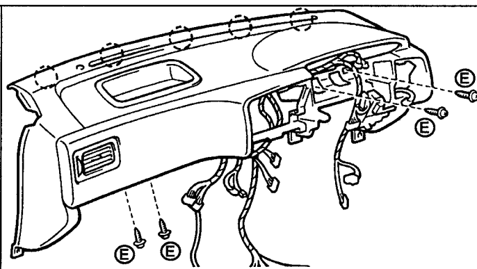
Снятие и установка панели приборов (тип 1).
