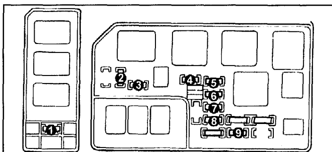
Возможный вариант монтажного блока №2 и блока плавких вставок (левая часть моторного отсека).
