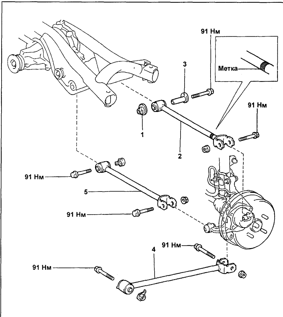
Снятие рычагов задней подвески. 1 - шайба, 2 - поперечный рычаг №2, 3 - регулировочная втулка, 4 - продольный рычаг, 5 - поперечный рычаг №1.
