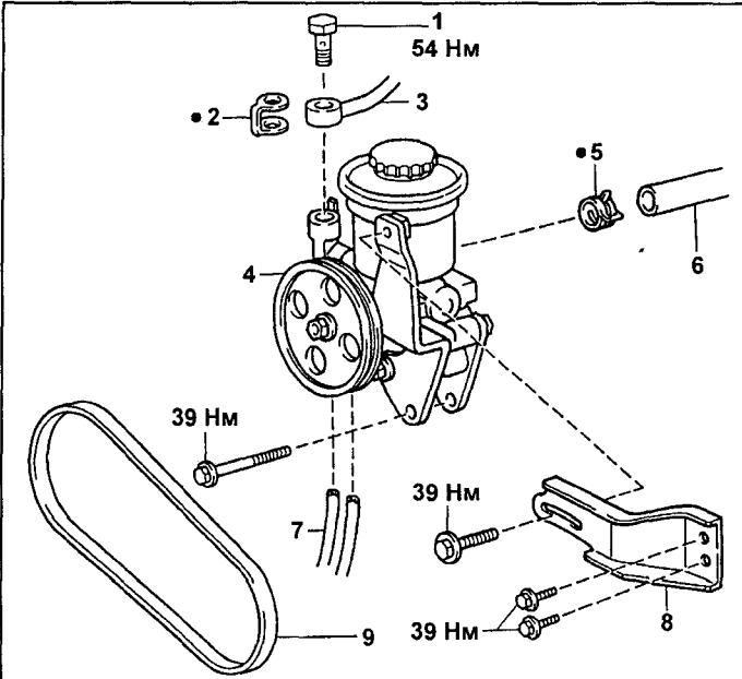
Снятие насоса усилителя рулевого управления (4A-FE, 7A-FE). 1 - штуцерный болт, 2 - прокладка, 3 - нагнетательный трубопровод, 4 - насос в сборе, 5 - хомут, 6 - возвратный трубопровод, 7 - вакуумные трубки, 8 - кронштейн крепления насоса, 9 - ремень привода насоса.
