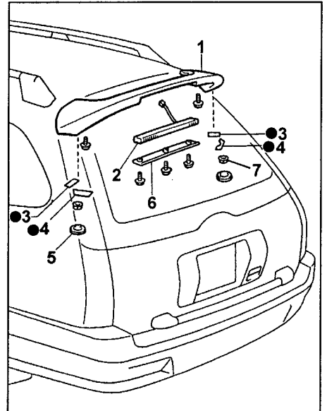
Задний спойлер. 1 - задний спойлер, 2 - дополнительный стоп сигнал, 3 - передняя проставка, 4 - боковая проставка, 5 - декоративная заглушка, 6 - нижняя крышка крепления дополнительного стоп сигнала, 7 - гайка.
