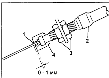
A241H (7A-FE), A245E. 1 - стопор, 2 - внешний трос, 3 - регулировочные гайки, 4 - чехол.
