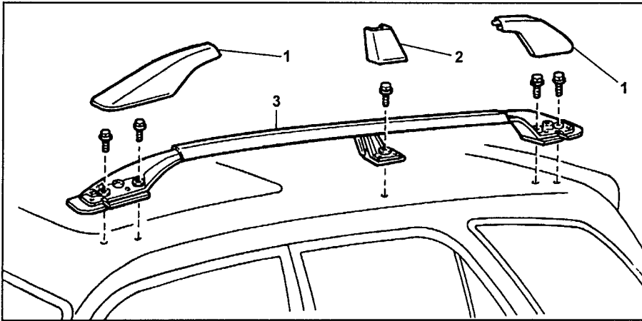
Багажник. 1 - боковые декоративные крышки багажника, 2 - центральная декоративная крышка багажника, 3 - стойка багажника.
