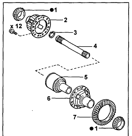
Ведущая шестерня главной передачи раздаточной коробки (с вязкостной муфтой). 1 - подшипник, 2 - правая чашка ведущей шестерни главной передачи, 3 - стопорное кольцо, 4 - промежуточный вал полуосевых шестерен №2, 5 - вязкостная муфта в сборе, 6 - левая чашка ведущей шестерни главной передачи, 7 - ведущая шестерня главной передачи.
