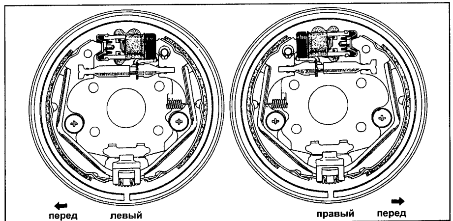
Схема установки деталей задних барабанных тормозов (модели до 1996 г.).
