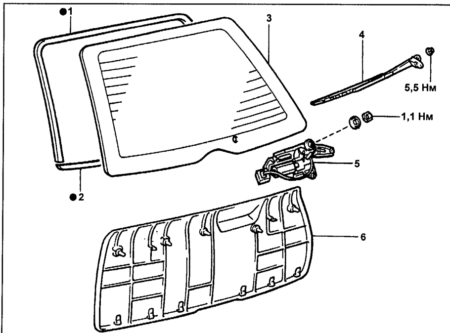
Стекло двери задка. 1 - верхний молдинг стекла двери задка, 2 - нижний молдинг стекла двери задка, 3 - стекло двери задка, 4 - поводок стеклоочистителя, 5 - электродвигатель стеклоочистителя, 6 - внутренняя нижняя накладка двери задка.
