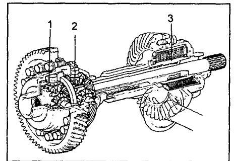
Схема полного привода с вязкостной муфтой. 1 - межколесный дифференциал, 2 - межосевой дифференциал, 3 - вязкостная муфта.
