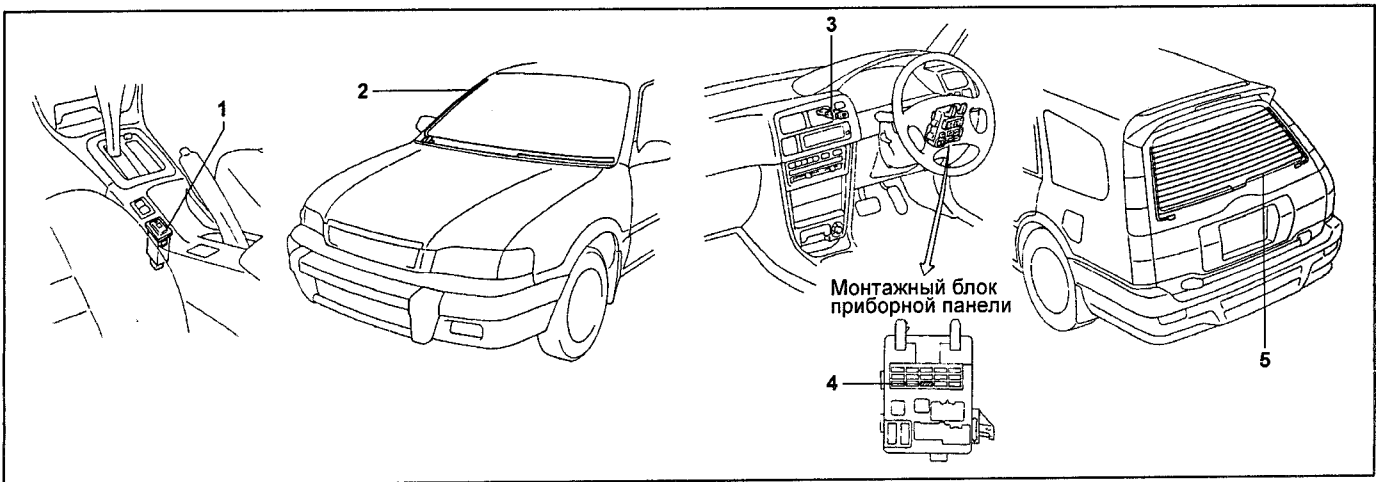
1 - выключатель антиобледенителя щеток, 2 - антиобледенитель щеток, 3 - выключатель обогревателя стекла двери задка, 4 - предохранитель DEFOG 30A, 5 - обогреватель стекла двери задка.
