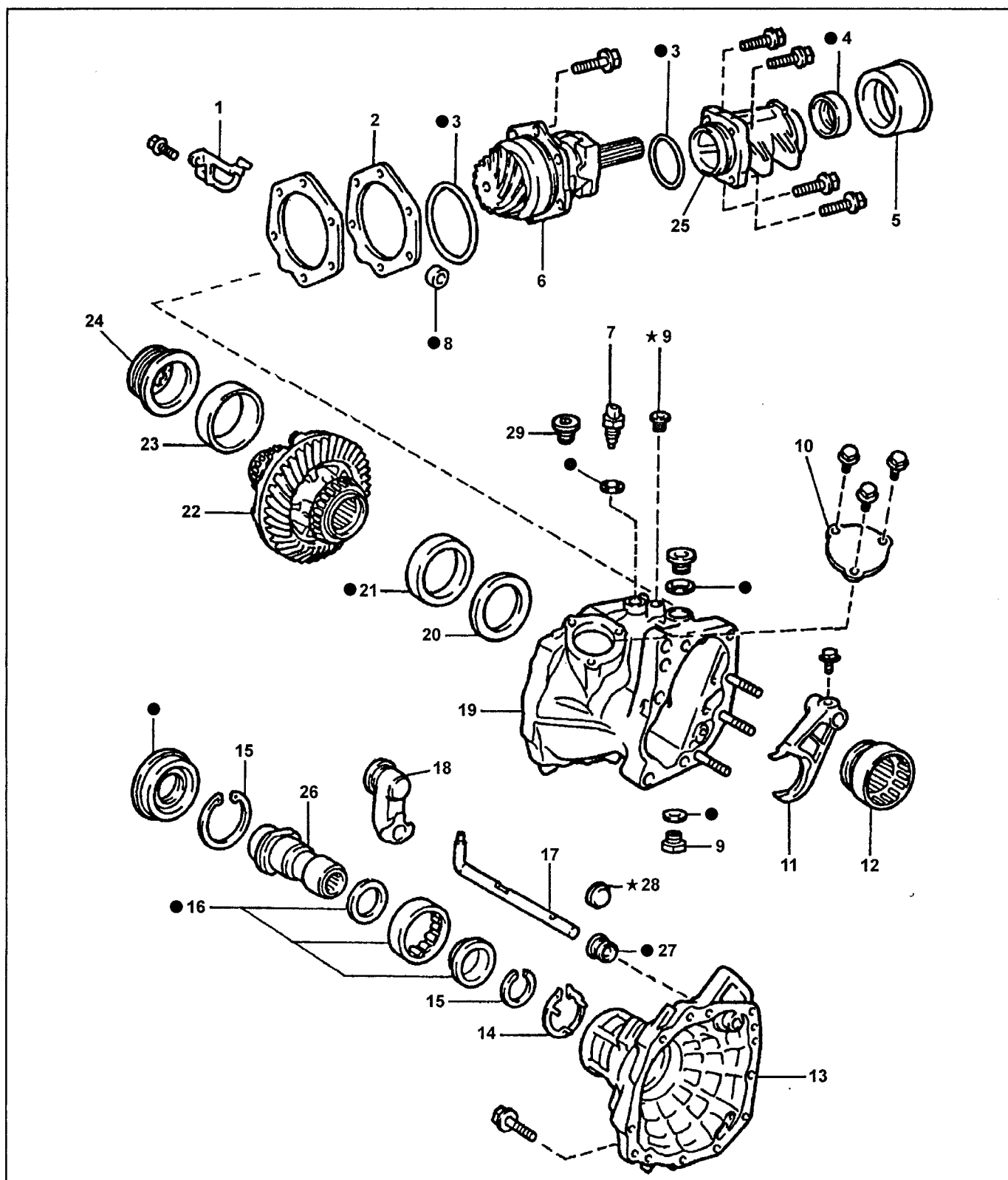
Раздаточная коробка. 1 - масляная трубка раздаточной коробки, 2 - регулировочная прокладка, 3 - кольцевое уплотнение, 4 - сальник, 5 - пыльник, 6 - держатель подшипников ведомой шестерни, 7 - датчик индикатора системы блокировки межосевого дифференциала (с механической блокировкой), 8 - втулка, 9 - пробка, 10 - крышка смотрового отверстия раздаточной коробки, 11 - вилка включения блокировки межосевого дифференциала (с механической блокировкой), 12 - муфта блокировки межосевого дифференциала (с механической блокировкой), 13 - крышка картера раздаточной коробки, 14 - стопорная пластина регулировочной гайки, 15 - стопорное кольцо, 16 - опорный подшипник промежуточного вала полуосевых шестерен, 17 - шток вилки включения блокировки межосевого дифференциала (с механической блокировкой), 18 - пыльник (с механической блокировкой), 19 - картер раздаточной коробки, 20 - шайба, 21 - наружное кольцо подшипника, 22 - вал ведущей шестерни главной передачи в сборе (с механической блокировкой), 23 - наружное кольцо подшипника, 24 - регулировочная гайка, 25 - удлинитель картера раздаточной коробки, 26 - держатель промежуточного вала полуосевых шестерен, 27 - сальник (с механической блокировкой), 28 - пробка (с вязкостной муфтой), 29 - заглушка (с вязкостной муфтой).
