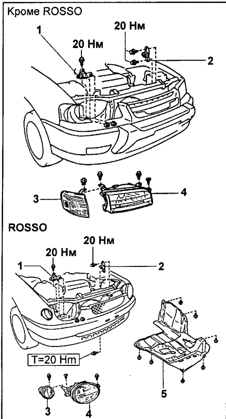
Передние датчики системы безопасности. 1 - правый датчик, 2 - левый датчик, 3 - указатель поворота, 4 - фара, 5 - защита двигателя.
