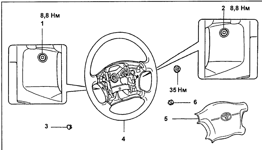
Снятие и установка подушки безопасности водителя (модели с 1996 года, SV Touring). 1, 2 - установочный болт накладки, 3, 6 - крышка рулевого колеса, 4 - рулевое колесо, 5 - накладка рулевого колеса.
