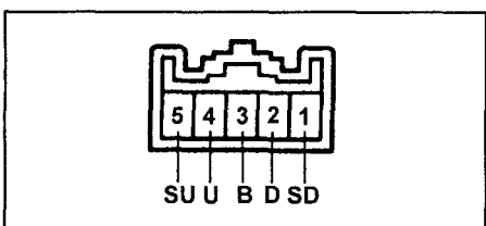
Задние двери (тип 2)
