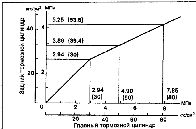
График работы регулятора давления (модели 4WD с 1996 г.).
