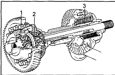
Схема полного привода с вязкостной муфтой. 1 - межколесный дифференциал, 2 - межосевой дифференциал, 3 - вязкостная муфта.
