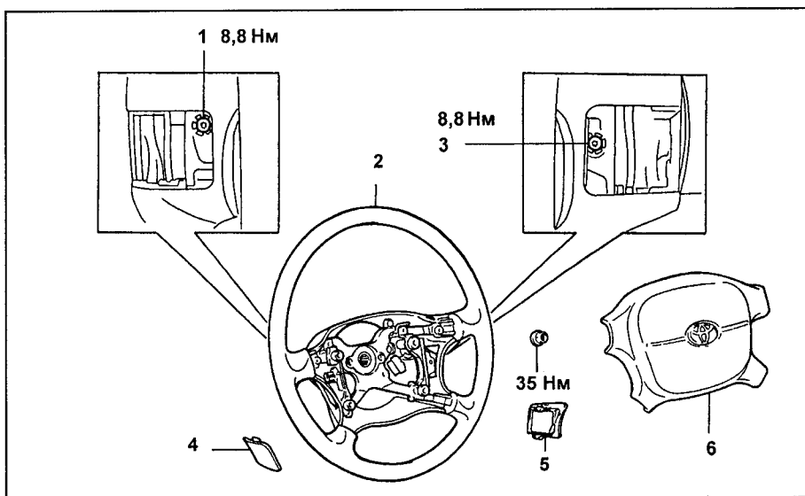
Снятие и установка подушки безопасности водителя (модели с 1996 года, BZ Touring). 1, 3 - установочный болт накладки, 2 - рулевое колесо, 4, 5 - крышка рулевого колеса, 6 - накладка рулевого колеса.
