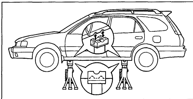
Точки установки лап подъемника.
