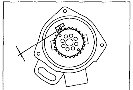
Датчик NE (4A-GE).
