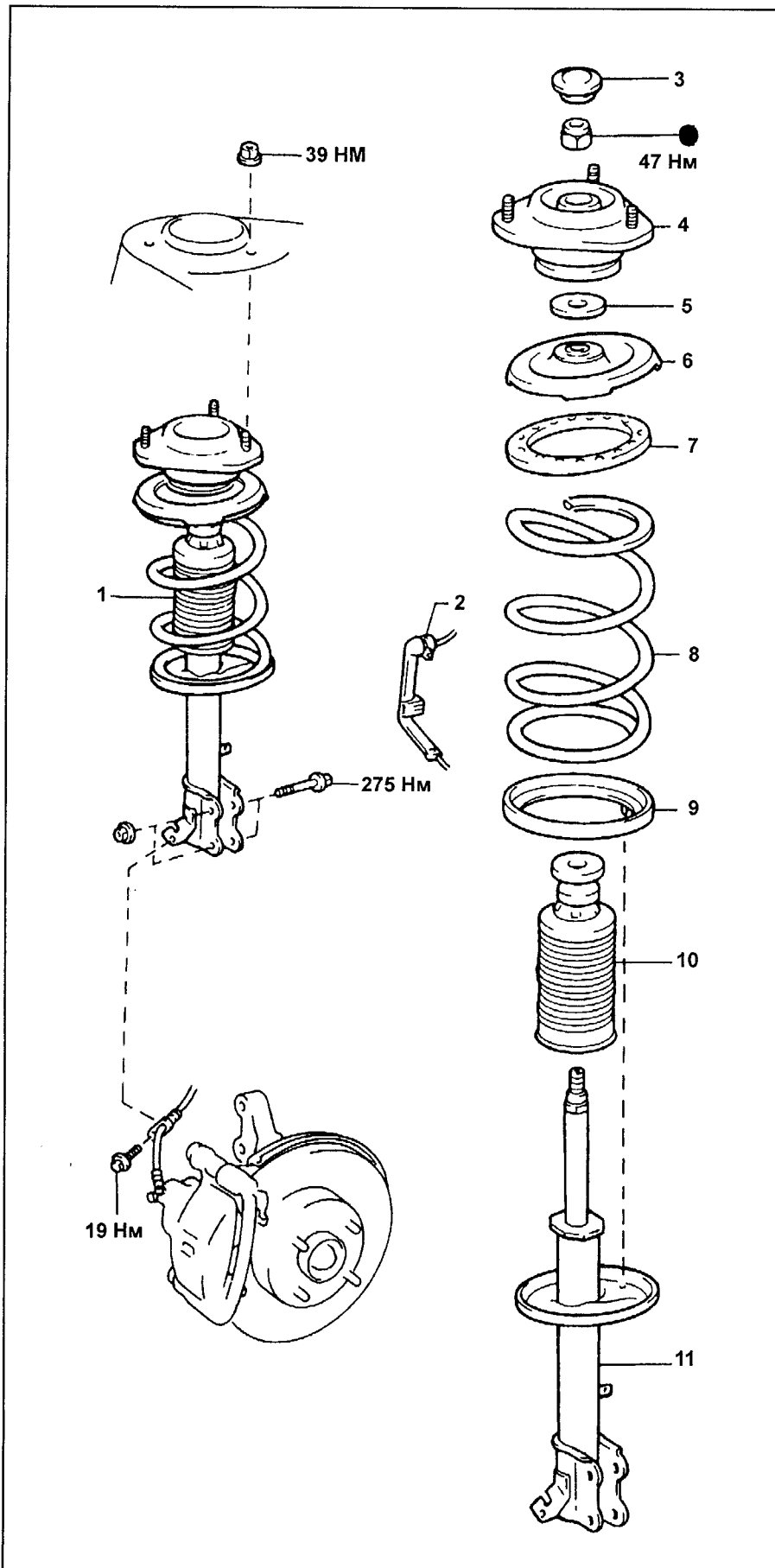
Стойка передней подвески. 1 - стойка передней подвески в сборе, 2 - кронштейн провода датчика частоты вращения (ABS), 3 - заглушка, 4 - верхняя опора стойки, 5 - уплотнение, 6 - верхнее седло пружины, 7 - верхний виброизолятор, 8 - пружина, 9 - нижний виброизолятор, 10 - ограничитель хода сжатия, 11 - стойка передней подвески.
