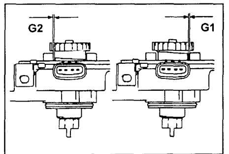
Датчик G (4A-GE).
