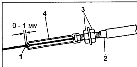
A241H (4A-FE). 1 - стопор, 2 - внешний трос, 3 - регулировочные гайки, 4 - гибкий чехол.
