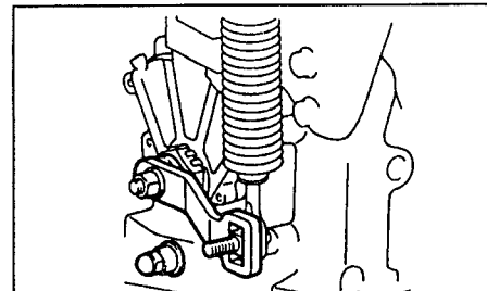
A241H (4A-FE). 1 - стопор, 2 - внешний трос, 3 - регулировочные гайки, 4 - гибкий чехол.
