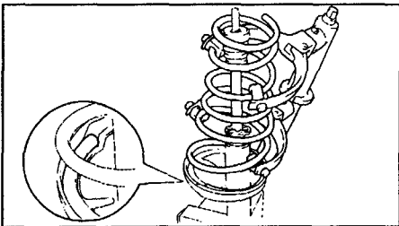
Стойка задней подвески. 1 - крышка, 2 - стойка стабилизатора поперечной устойчивости, 3 - стойка задней подвески в сборе, 4 - фиксатор, 5 - датчик частоты вращения (ABS), 6 - втулка, 7 - верхняя опора стойки, 8 - ограничитель хода сжатия, 9 - пружина, 10 - нижнее седло пружины, 11 - стойка задней подвески.
