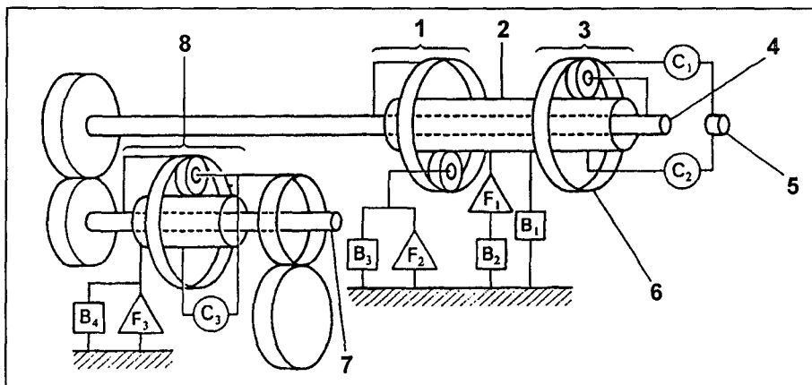
Схема АКПП (А241Н, А245Е). 1 - задний планетарный ряд, 2 - солнечные шестерни переднего и заднего планетарных рядов, 3 - передний планетарный ряд, 4 - промежуточный вал, 5 - входной вал, 6 - эпицикл, 7 - вал ведущей шестерни главной передачи, 8 - понижающий планетарный ряд.
