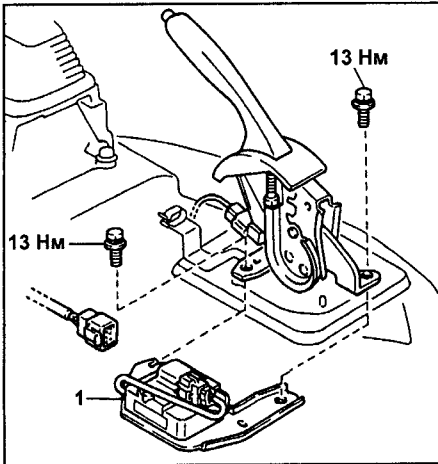
Снятие датчика замедления. 1 - датчик замедления.
