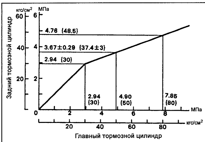
График работы регулятора давления (модели 2WD с 1996 г. (4A-GE)).
