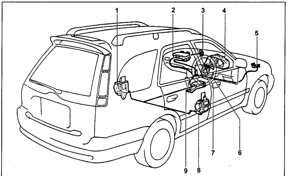
Система безопасности (модели с 1998 года). 1 - преднатяжитель левого ремня безопасности, 2 - подушка безопасности пассажира, 3 - левый передний датчик столкновения, 4 - комбинация приборов (индикатор SRS), 5 - правый передний датчик столкновения, 6 - спиральный провод, 7 - накладка рулевого колеса, 8 - преднатяжитель ремня безопасности водителя, 9 - центральный датчик системы безопасности.
