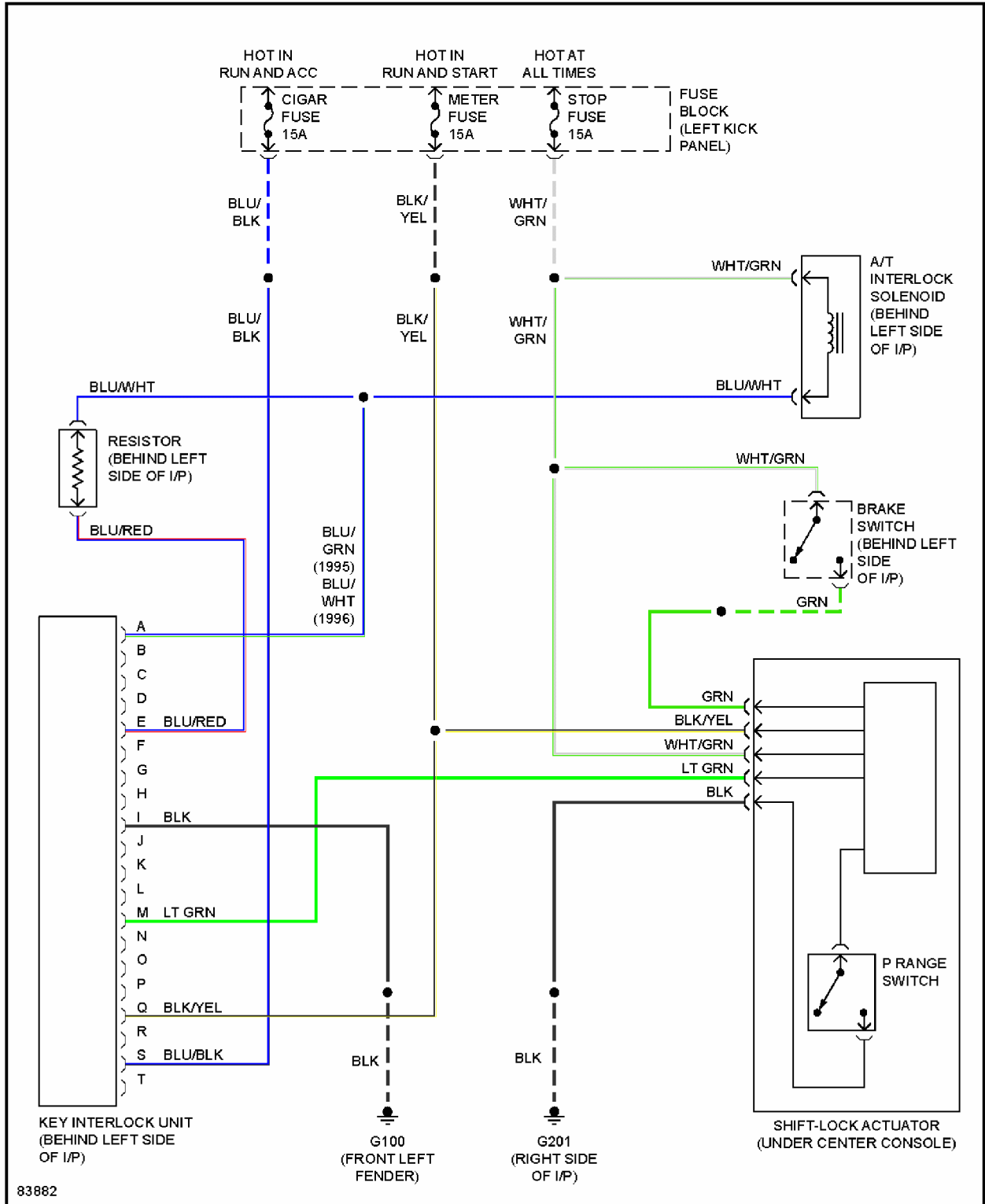
Fig. 25: Shift Interlock Circuit
