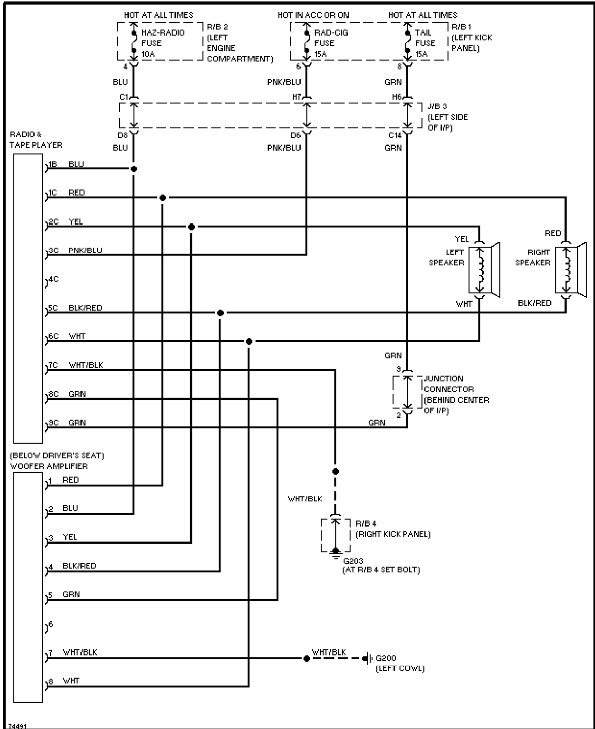
Radio Circuits
