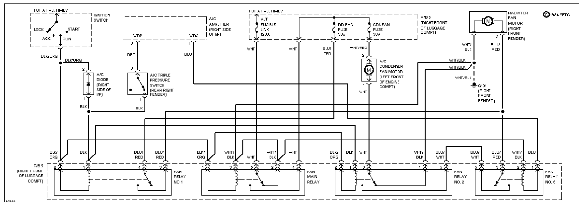
Cooling Fan Circuit
